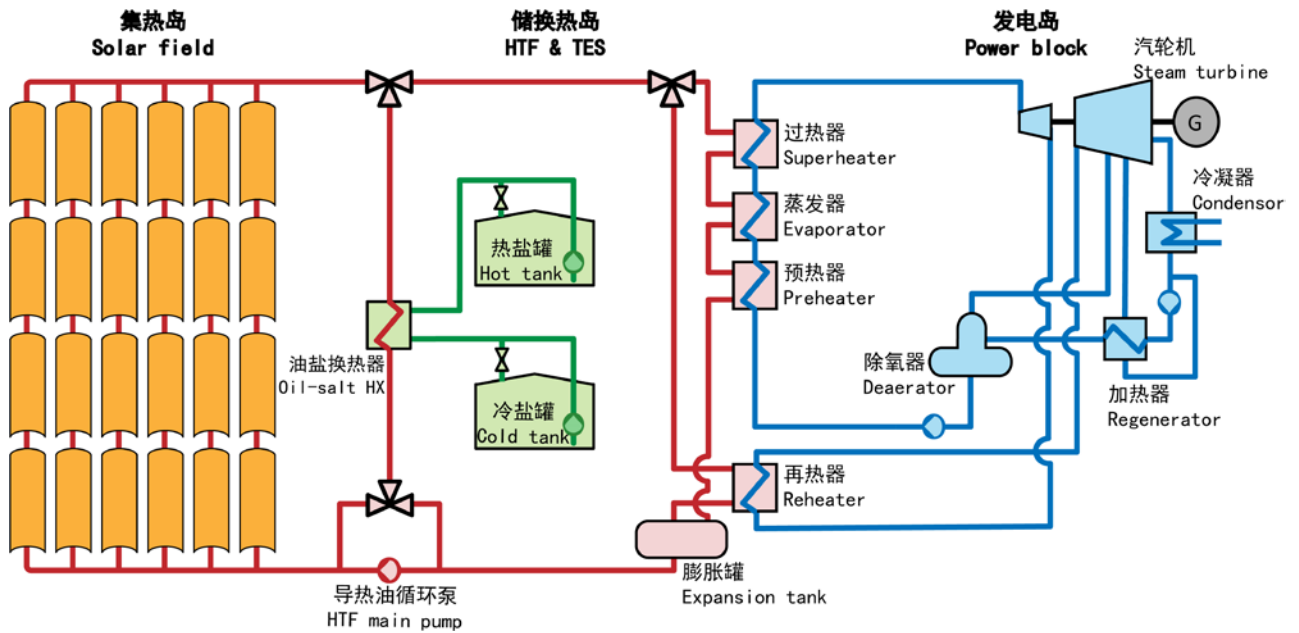
图：导热油槽式太阳能热发电系统（常规流程）示意图（图片来源：龙腾光热）
