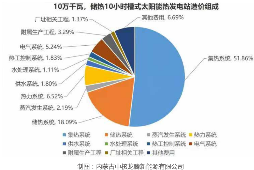
图：我国 10 小时储热 100MW 导热油槽式电站投资组成
